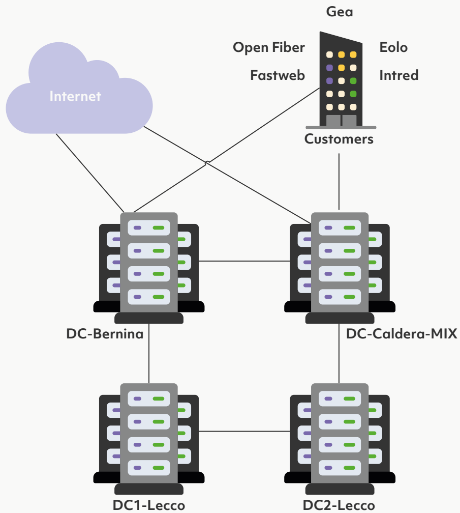
Figura 1 Schema di principio servizio Layer 3
